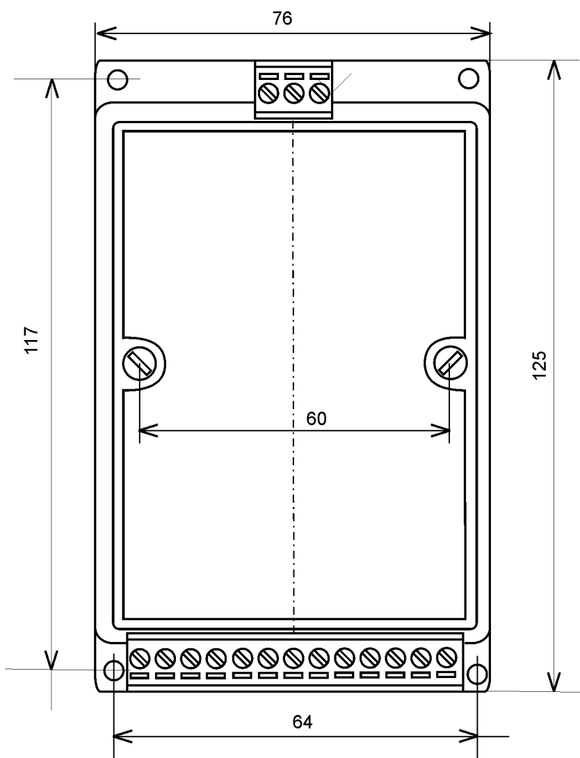
Рис. 3.1. Габаритный чертеж и присоединительные размеры источника пи-
