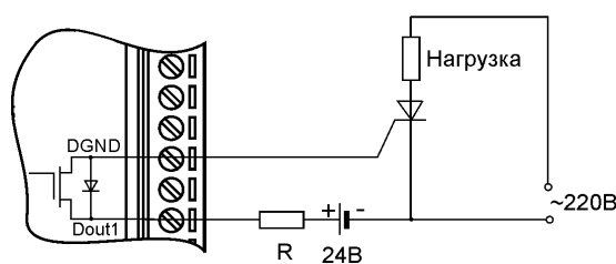
Рис. 6.8. Обратите внимание, что при отсутствии питания модуля симистор выключен, что соответствует требованиям к аварийным режимам оборудования. Однако такая схема не позволяет подключить симисторы
