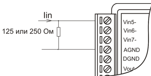
Рис. 6.7. Пример подключения шунтирующего резистора на 13-й одиночный канал модуля NL-8AI для измерения тока в диапазоне \pm 20 мА.
