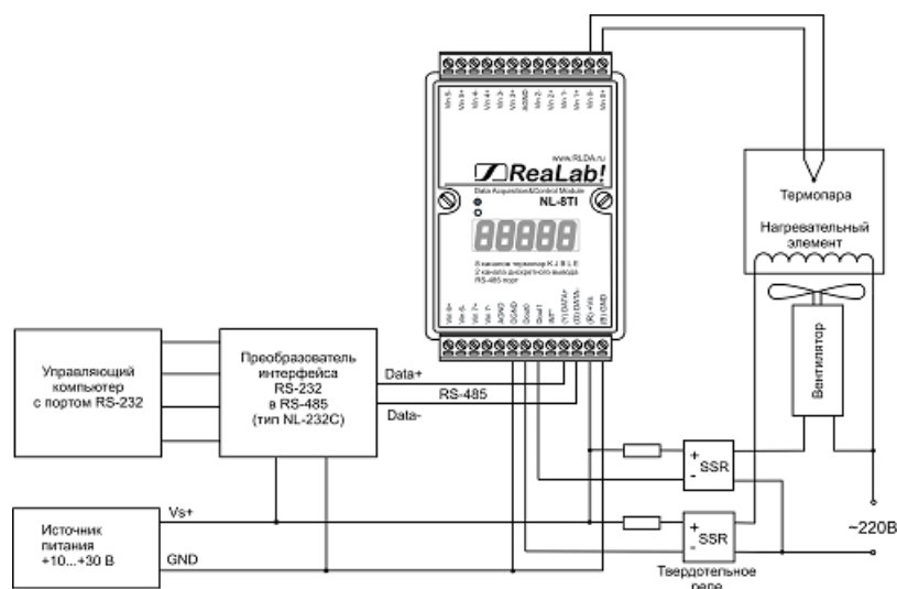
Рис. 6.11. Применение модуля для стабилизации температуры. Управляющий компьютер и преобразователь интерфейса после конфигурирования модуля могут быть исключены из системы
