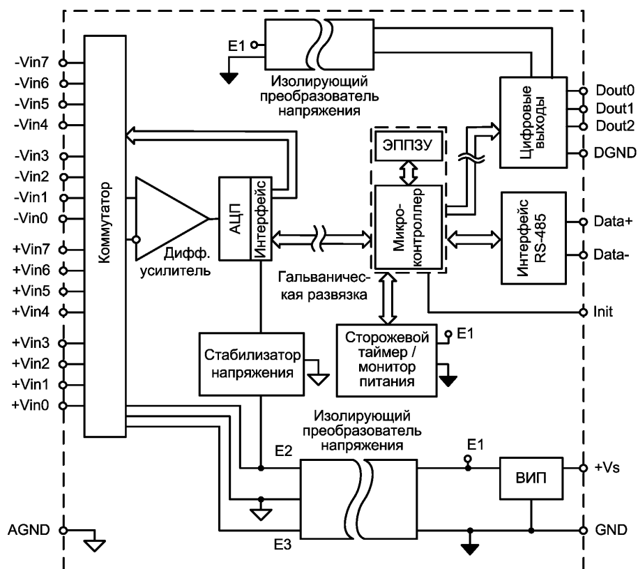
Рис. 5.3. Структурная схема модуля NL-8AI в режиме одиночных входов. В режиме дифференциальных входов Vin0...Vin7 являются неинвертирующими входами каналов с 0-го по 7-й, входы Vin8...Vin15 являются инвертирующими входами каналов с 0-го по 7-й. Например, входом 0-го дифференциального канала являются выводы +Vin0 и -Vin8, 1-го канала - входы +Vin1 и -Vin9 и т.д.
