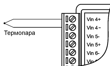
Рис. 6.5 . Подключение термопары к каналу 4 модуля.
