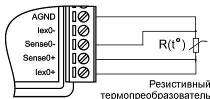
Рис. 6.14. Четырехпроводное подключение резистивного термопреобразователя к модулю
