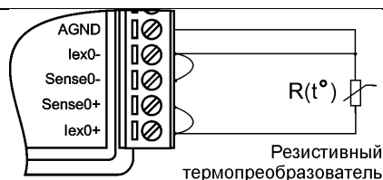
Рис. 6.13. Трехпроводное подключение резистивного термопреобразователя к модулю
