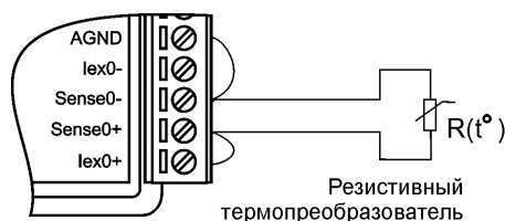
Рис. 6.12. Двухпроводное подключение резистивного термопреобразователя к модулю
