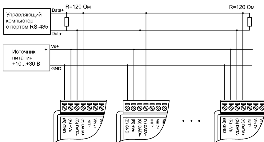
Рис. 6.15. Соединение нескольких модулей в сеть на основе интерфейса RS-485
