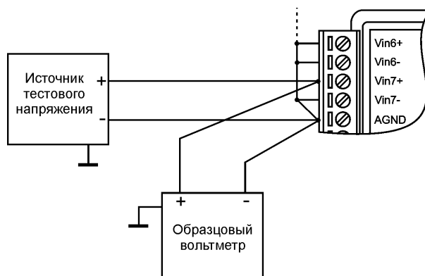
Рис. 5.4. Соединение приборов для юстировки модулей
