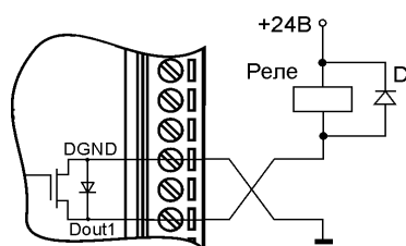
Рис. 6.9. Применение модуля для управления электромагнитным реле
