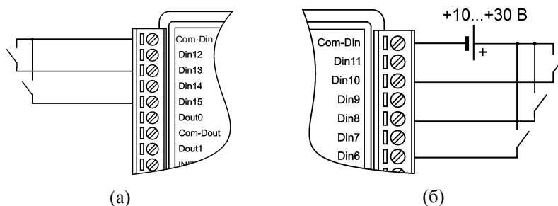
Рис. 5.6. Подсоединение контактов к модулю с входным каскадом типа «Сухой контакт» (а) и с входным каскадом типа логический вход («Мокрый контакт») (б)
