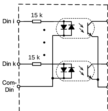
Рис. 4.7. Входной каскад типа логический вход («мокрый контакт») модулей NL-16DI и NL-16DO
