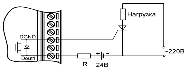
Рис. 5.9. Применение модуля для управления мощным тиристором
