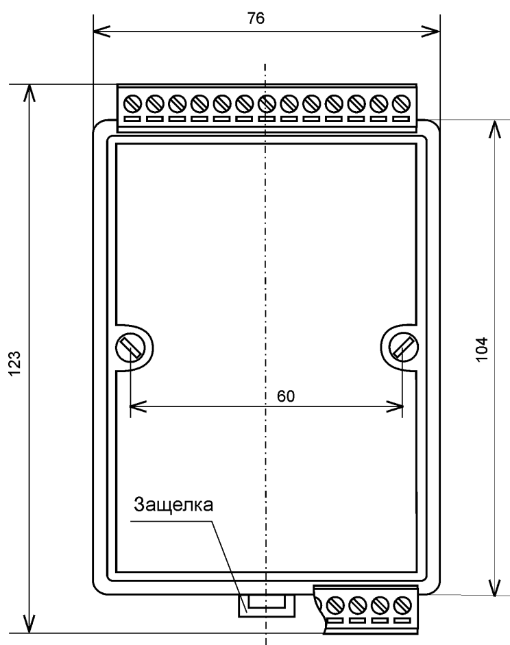
Рис. 2.5. Габаритный чертеж модуля.
