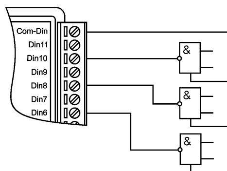
Рис. 5.7. Подсоединение источников сигналов с логическими уровнями
