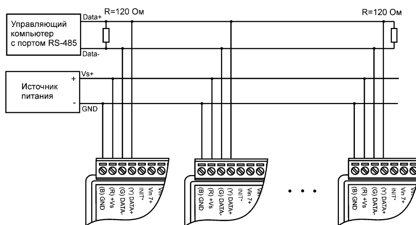
Рис. 5.12. Соединение нескольких модулей в сеть на основе интерфейса RS-485
