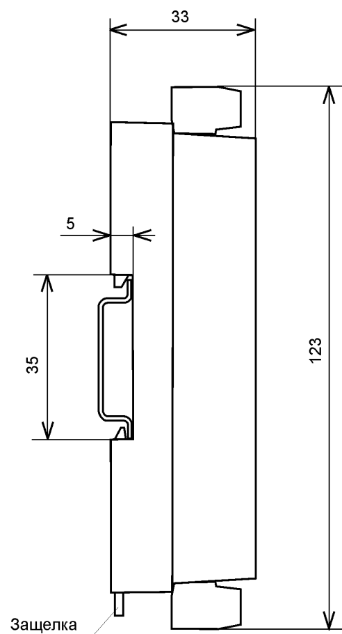
Рис. 2.6. Габаритный чертеж модуля с креплением к DIN-рейке. Планка для крепления к стене отсоединена. Вид сбоку.
