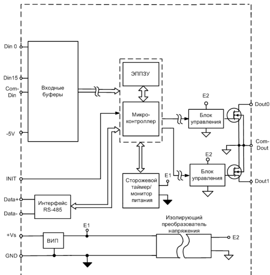
Рис. 4.1. Структурная схема модуля NL-16DI. Структуру входных каскадов см. на рис. 4.5 - рис. 4.7
