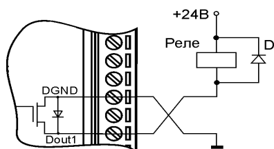
Рис. 5.10. Применение модуля для управления электромагнитным реле
