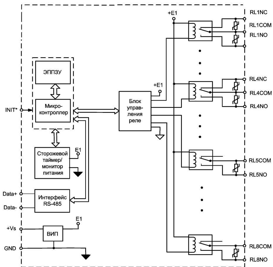
Рис. 4.4. Структурная схема модуля NL-8R. Обозначения: COM - "Common" - "общий", "C" - "Closed" - постоянно замкнутый, "O" - "Open" - постоянно открытый
