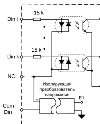
Рис. 4.5. Входной каскад типа "сухой контакт" модуля NL-16DI
