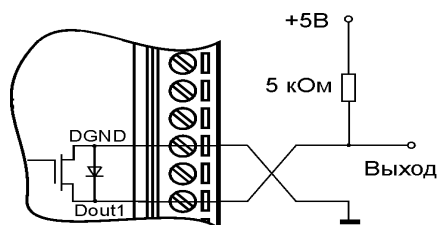
Рис. 5.11. Получение логических уровней напряжения на выходах модуля
