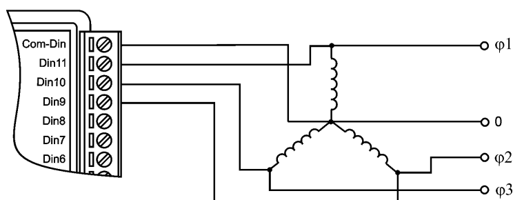
Рис. 5.8. Контроль обрыва фазы в подводящих цепях 220/380 В трехфазного двигателя с помощью модуля NL-16HV
