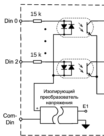
Рис. 4.6. Входной каскад в модуле NL-16DO ("сухой контакт")
