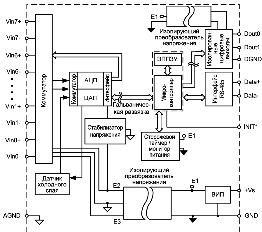
Рис. 5.1. Структурная схема модуля NL-8TI, взрывозащищённого исполнения
