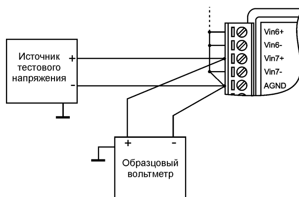
Рис. 5.4. Соединение приборов для юстировки модулей
