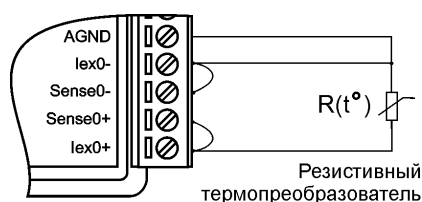
Рис. 6.11. Трехпроводное подключение резистивного термопреобразователя к модулю
