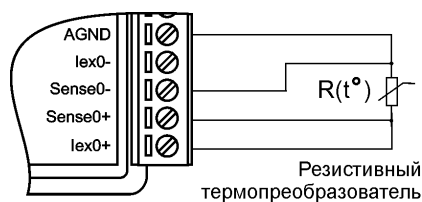
Рис. 6.12. Четырехпроводное подключение резистивного термопреобразователя к модулю
