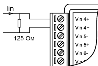
Рис. 6.7. Подключение резистора 125 Ом для измерения тока I_{in} .
