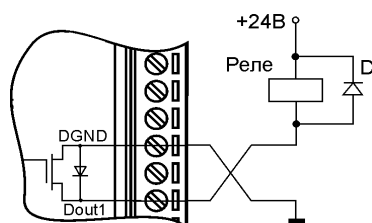
Рис. 6.8. Применение модуля для управления электромагнитным реле
