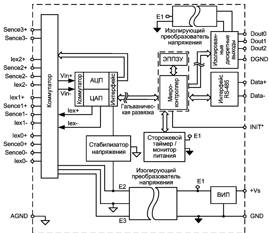
Рис. 5.2. Структурная схема модуля NL-4RTD, взрывозащищённого исполнения
