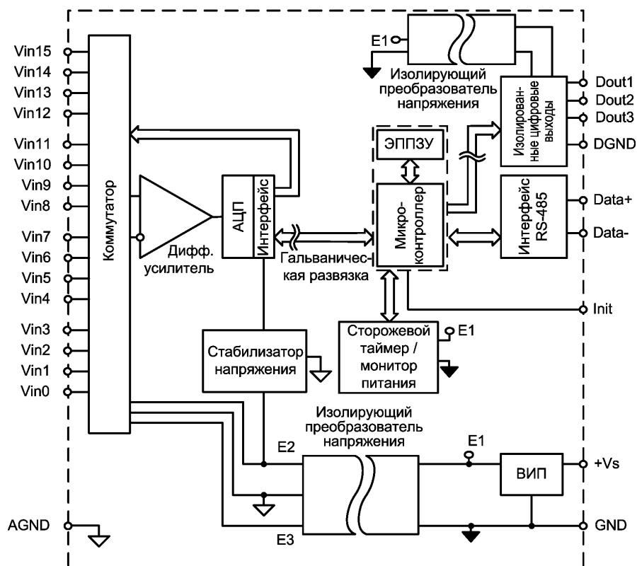
Рис. 5.3. Структурная схема модуля NL-8AI, взрывозащищённого исполнения, в режиме одиночных входов. В режиме дифференциальных входов Vin0...Vin7 являются неинвертирующими входами каналов с 0-го по 7-й, входы Vin8...Vin15 являются инвертирующими входами каналов с 0-го по 7-й. Например, входом 0-го дифференциального канала являются выводы +Vin0 и -Vin8, 1-го канала - входы +Vin1 и -Vin9 и т.д.
