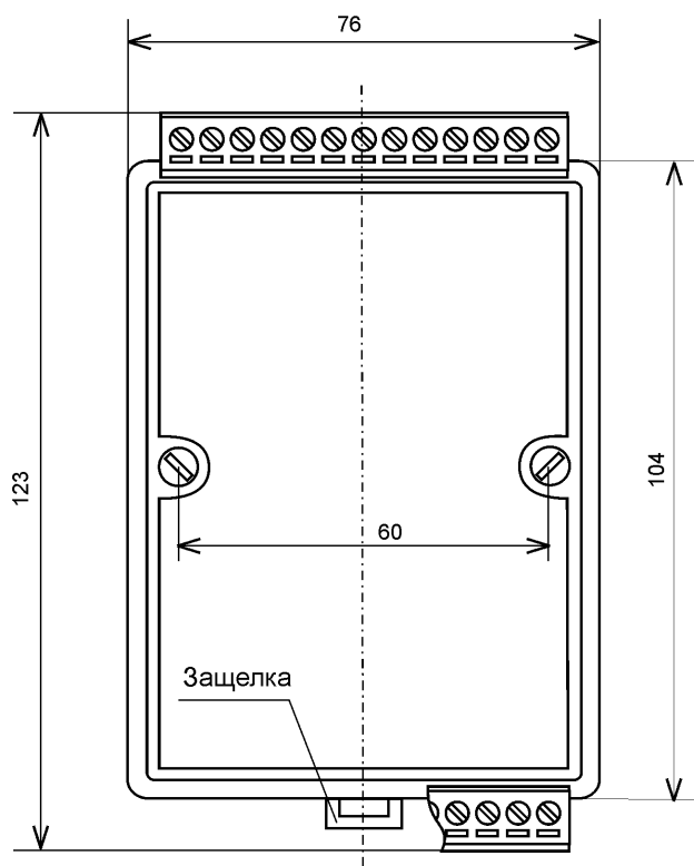
Рис. 2.4. Габаритный чертеж модуля.
