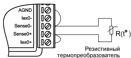
Рис. 6.10. Двухпроводное подключение резистивного термопреобразователя к модулю
